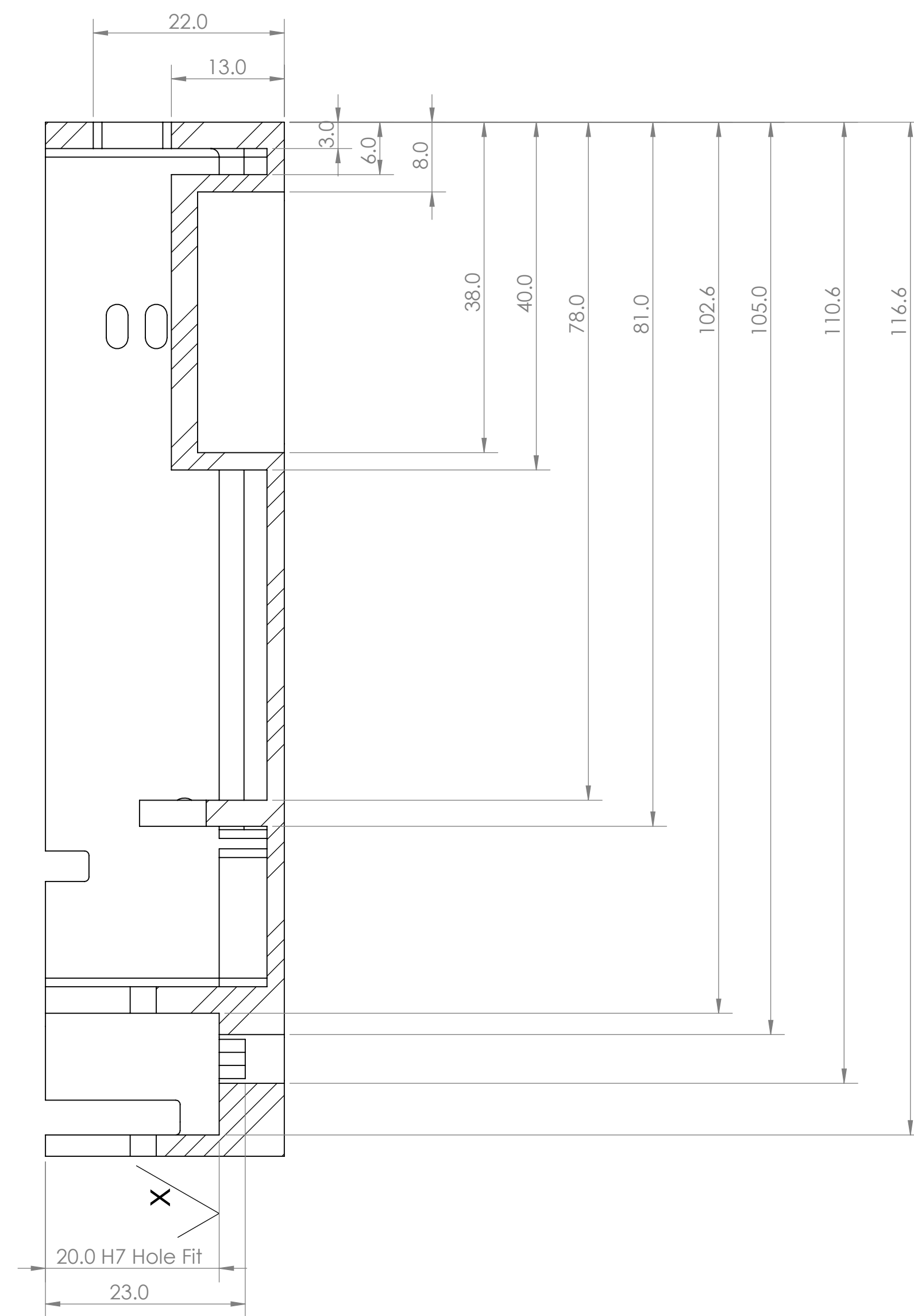
SECTION A-A
